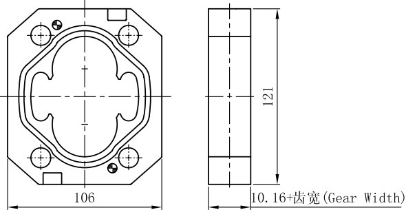
马达 (Motor)
