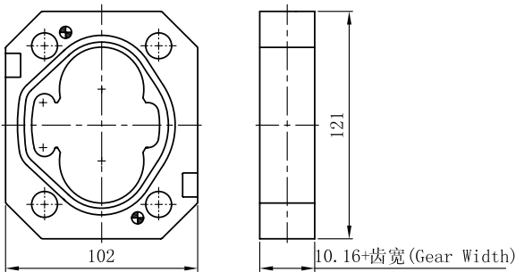
泵 (Pump)
